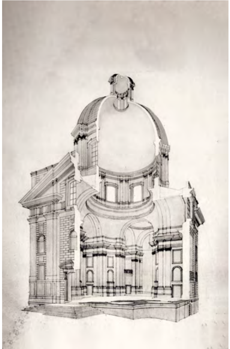
Praha, kostel sv. Františka z Assisi, řez
